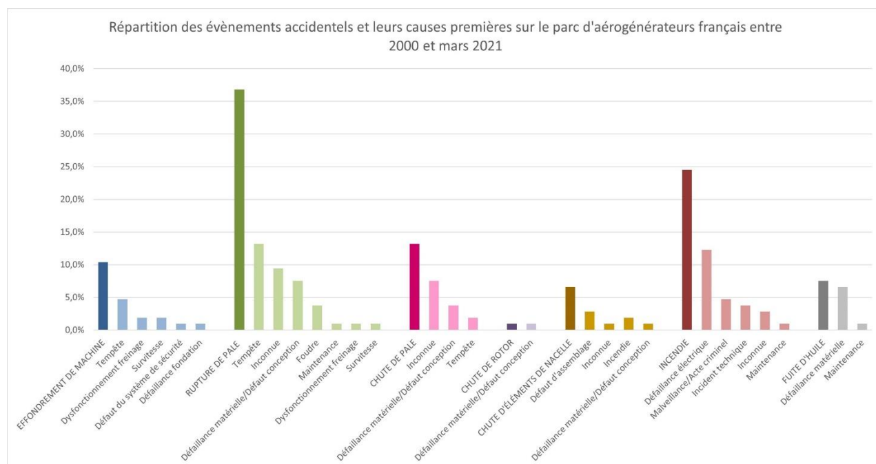
Figure 6 : Répartition des accidents et de leurs causes premières sur le parc éolien français entre 2000 et mars 2021 (source : ENCIS Environnement d'après le Guide technique, mai 2012)
