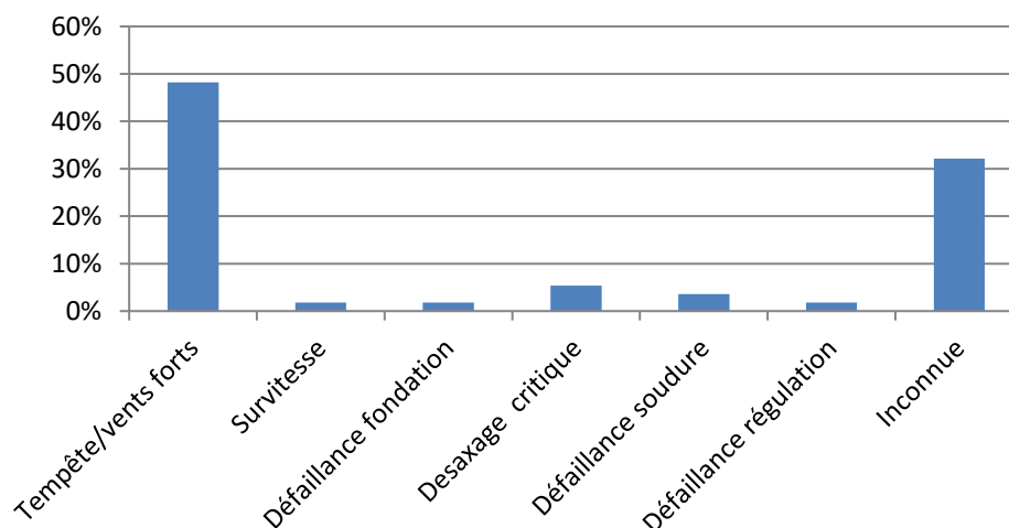
Figure 8 : Répartition des causes premières d'effondrement dans les accidents à l'international entre 2000 et 2011 (Source : Guide technique, mai 2012)
