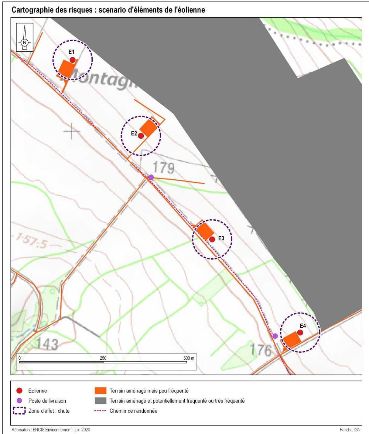
Carte 15 : Cartographie des risques – scenario : chute d'éléments (Source : ENCIS Environnement)
